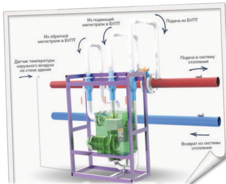
Блок управления потреблением тепла (БУПТ) — аналог автоматизированного насосного индивидуального теплового пункта, адаптированный для жилых многоквартирных домов.
