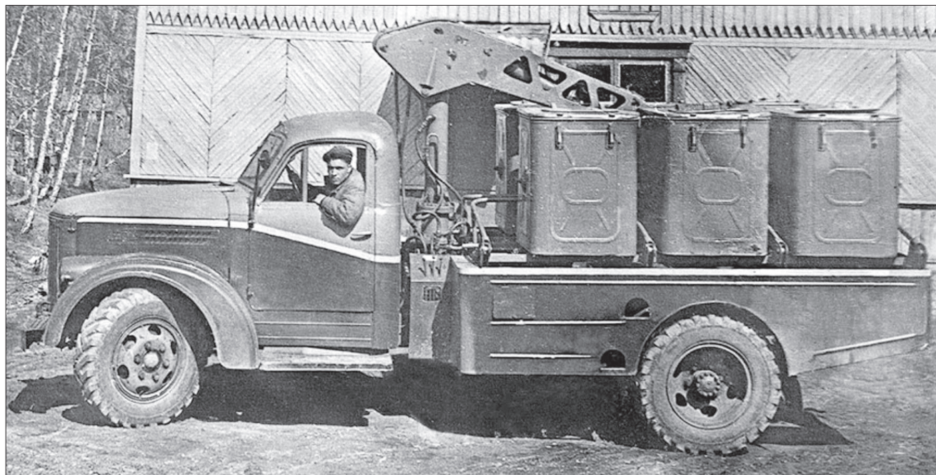
Вот так выглядел один из четырех озерских мусоровозов, смонтированных на шасси «Урал ЗИС-355М»
